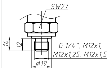
G1/4" DIN 3852
