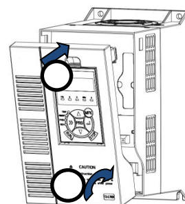
Рис.2-6 Снятие пластикового корпуса
