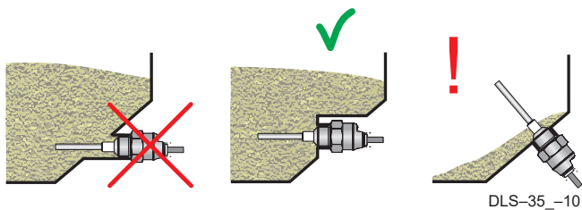
Монтаж в наклонную стенку резервуара
