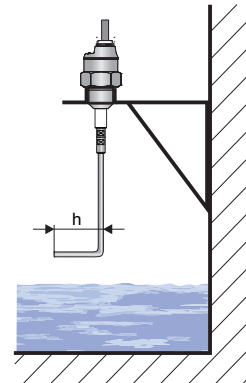
Изгибание конца электрода при считывании неизвестных жидкостей
