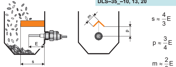
Монтаж защитной крышки
