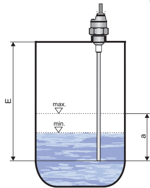
Регулирование уровня с помощью гистерезиса
