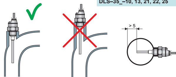
Монтаж датчика в трубу
