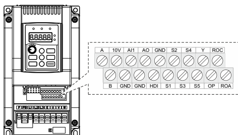
Рисунок 3-6. Схема расположения клемм цепей Управления преобразователя частоты SDI
