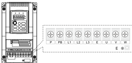
Рисунок 3-5. Схема цепей электропитания преобразователя частоты SDI
