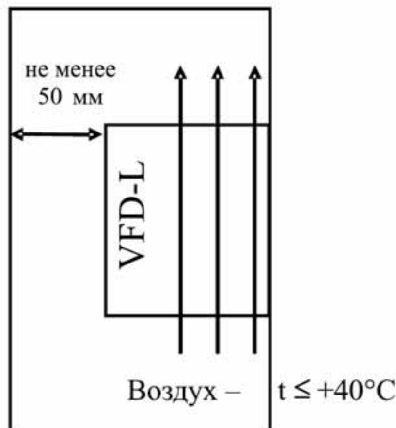
Вид сбоку
