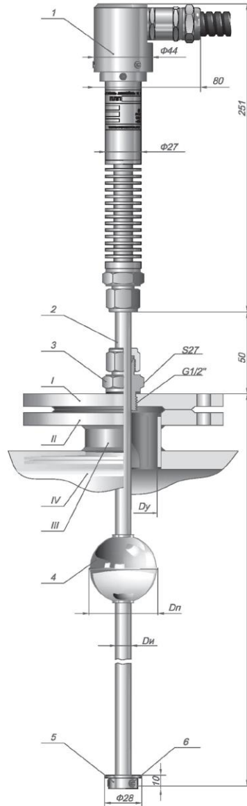
РИСУНОК В.6 Габаритно-установочный чертеж ПЛП1xxx-У-Т2
