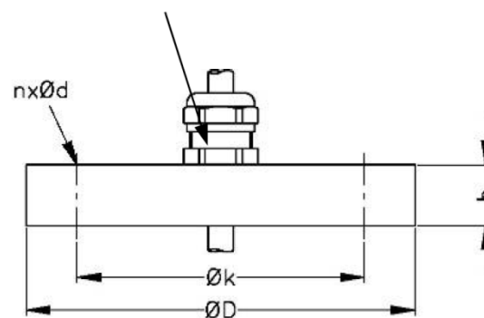
Кабельный ввод M16x1.5 под кабель Ø 4..11 мм
