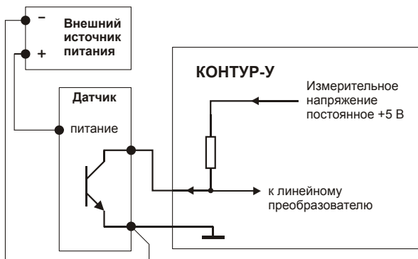
б) питание от внешнего источника
