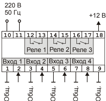
Схема электрическая подключения контроллера уровня универсального «Контур–У–Щ1»
