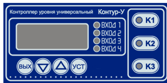
Лицевая панель контроллера «Контур-У-Щ1»
