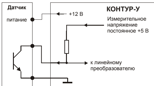
а) питание от прибора
