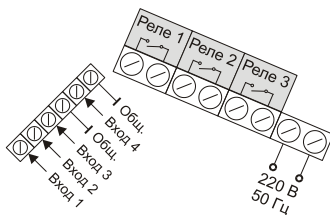
Схема электрическая подключения контроллера уровня универсального «Контур–У–Щ1»
