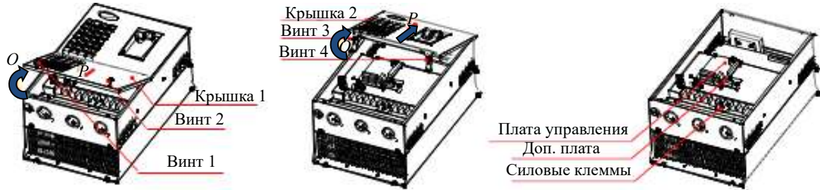
Рис.2-9 ITD...B3 (30~250 кВт)
