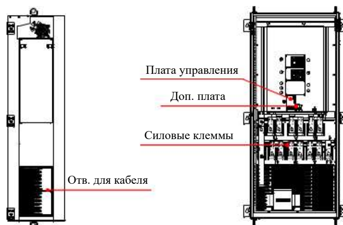
Рис.2-11 ITD...B3 (355~500 кВт)
