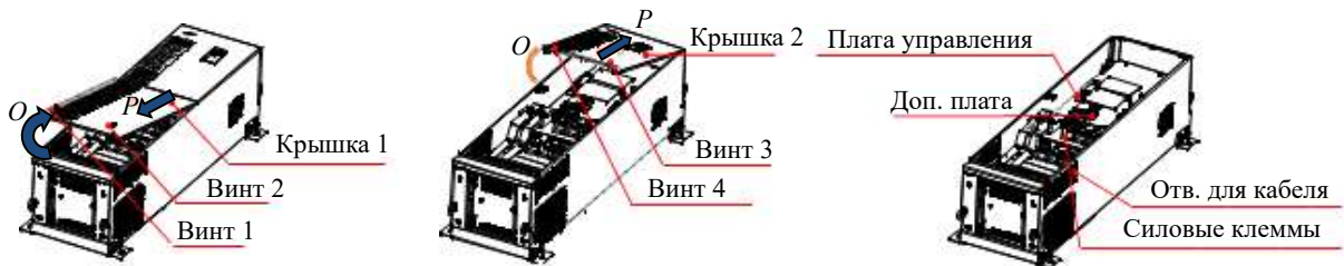
Рис.2-10 ITD...B3 (160~315 кВт)
