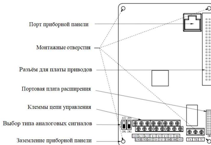
Рис. 3-20 Плата управления
