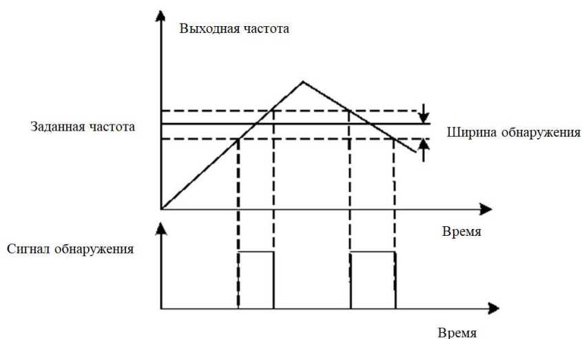
Рис.6-20 Схема обнаружения FAR
