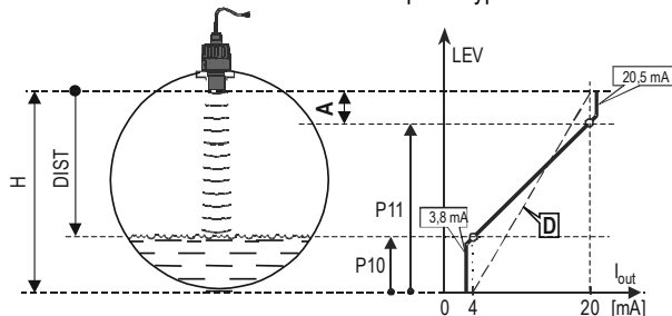
Измерение уровня
