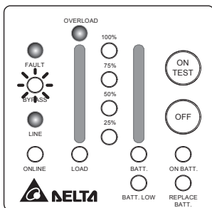
Рис. 3-14. Отказ вентилятора
