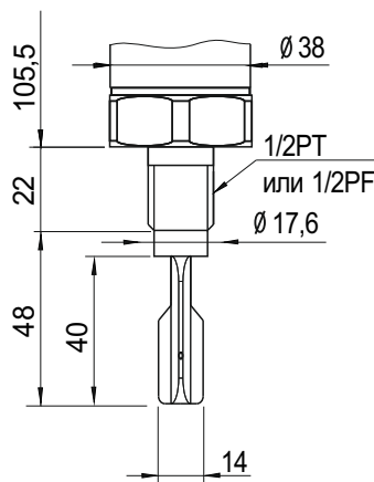
Версия с резьбой 1/2"
