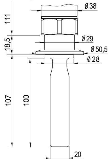
Версия с соединением Clamp DN40 зонд 100мм
