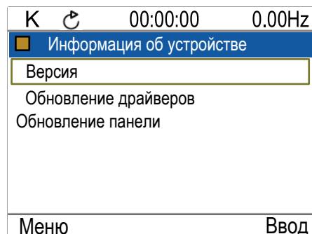
Рисунок 4.19 – Интерфейс «Устройство»
