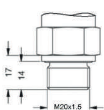
M20x1.5 DIN 3852
