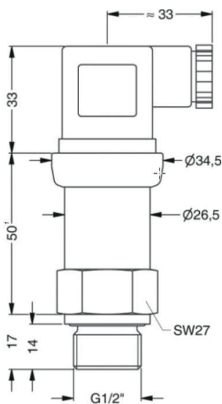
G1/2" DIN 3852
