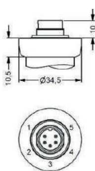
Разъем Binder 723, 5-конт. / IP 67
