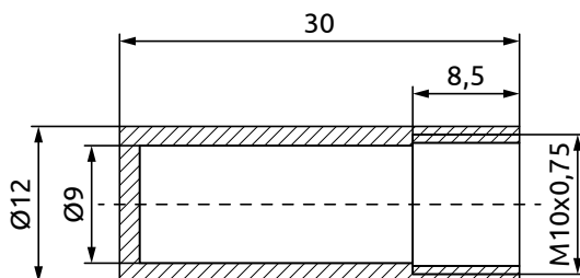
Рисунок А.3 - Габаритные размеры защитного колпачка HTE Cap.02
