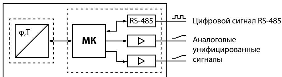
Рисунок 4 - Функциональная схема датчика
