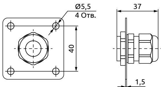
Рисунок А.1 - Габаритные размеры консоли HTE-HoldC
