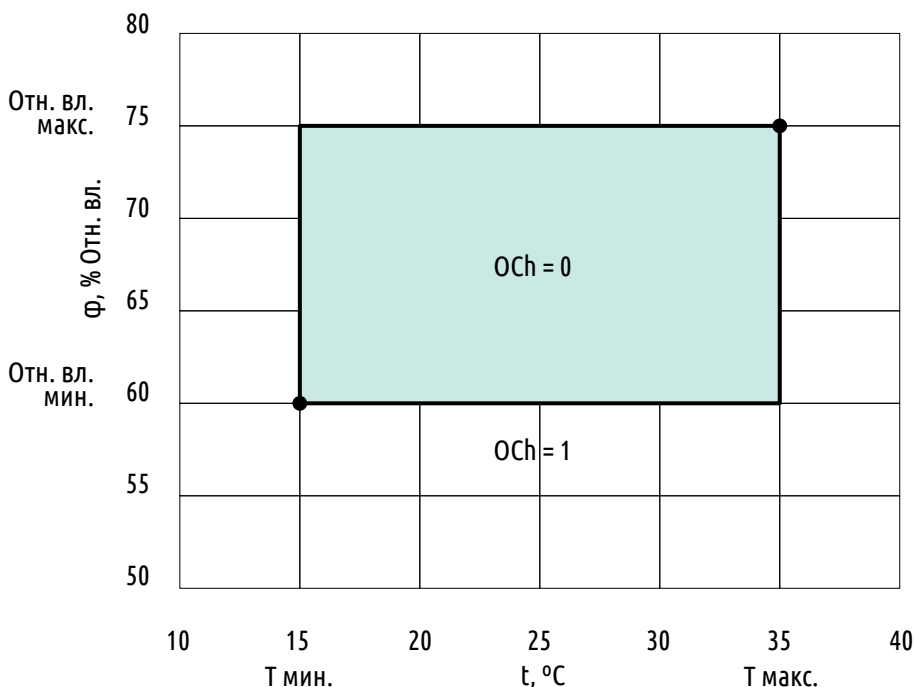
Рисунок 9 - Установка предельных значений относительной влажности и температуры
