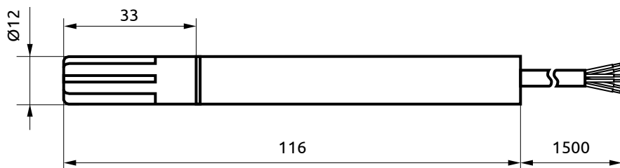
Рисунок 2 - Габаритные размеры HTE.PF с кабелем
