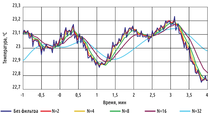
Рисунок 11 - Результат цифровой фильтрации показаний температуры (колпачок без фильтрующего материала)
