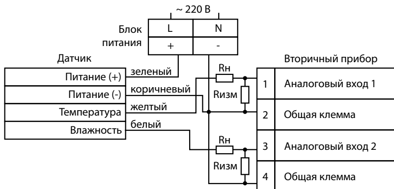
Рисунок 5 - Схема внешних электрических подключений датчиков HTE.PF-I42
