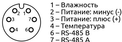
Рисунок 7 - Нумерация контактов разъема датчика HTE.PF-***M-(RS)
