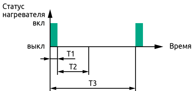
Рисунок 12 - Схема работы автоматического прогрева сенсора
