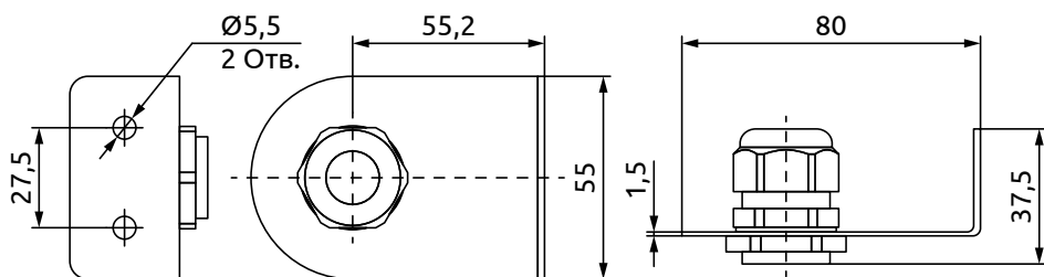
Рисунок А.2 - Габаритные размеры консоли HTE-HoldW
