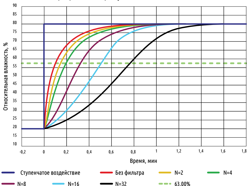
Рисунок 10 - Отклик датчика на ступенчатое воздействия с различными настройками цифровой фильтрации (колпачок без фильтрующего материала)
