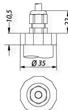
Каб. ввод PG7 с кабелем PVC 2 м / IP 67
