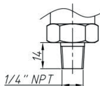
1/4"-18NPT
