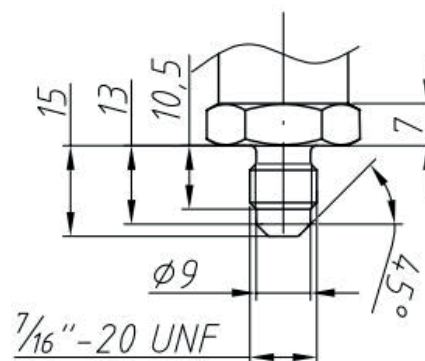
7/16-20"UNF
