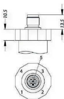
Разъем M12x1, 4-конт. / IP 67 или разъем M12x1 металлический, 4-конт. / IP 67
