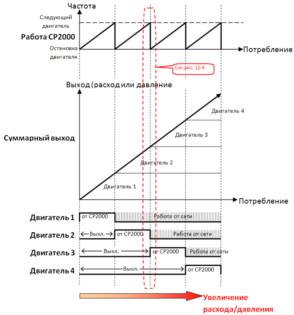
Рис. 12-3: Диаграмма работы каскадного управления с переменным мастером (ПИД) - Увеличение
