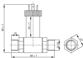
г) общий вид преобразователя, предназначенного для измерения дифференциального давления (с присоединительной резьбой G1/2) / d) general view of the transducer designed for differential pressure measurement (with connection thread G1/2) / г) дифференциалды қысымды өлшеуге арналған түрлендірілтің жалпы көрінісі (G1/2 жалғамалы бұрандамасымен бірге)
