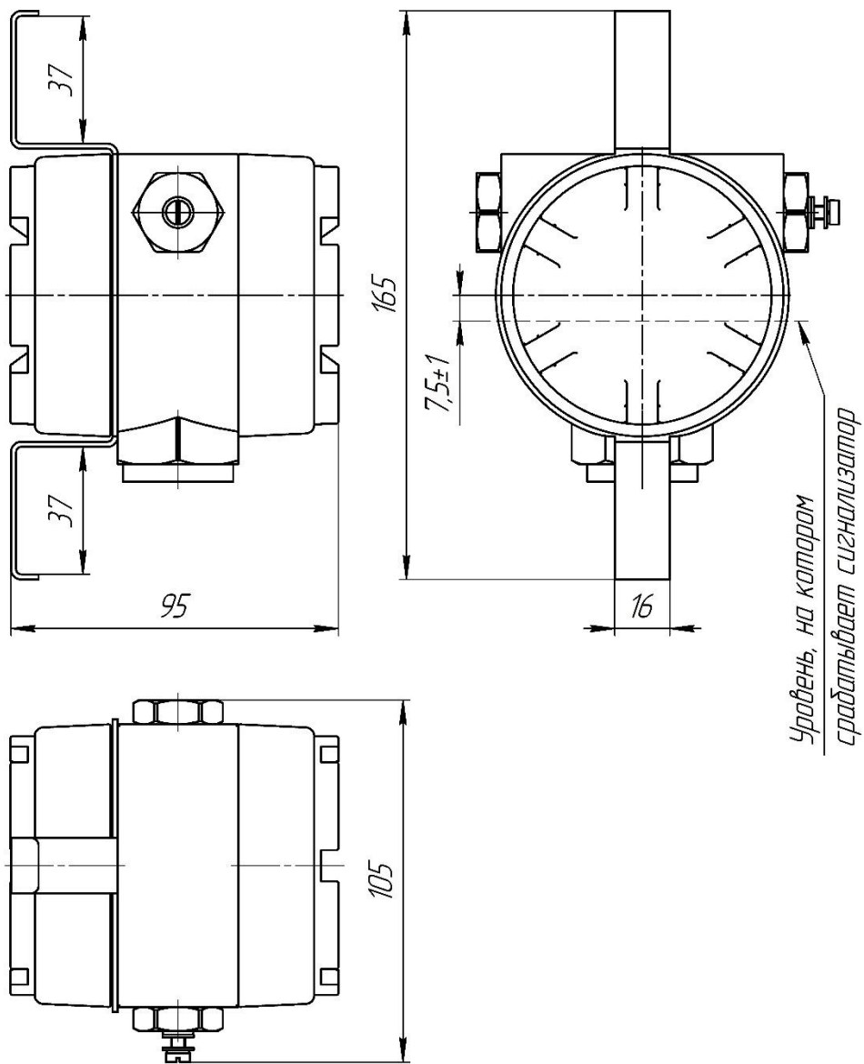
Рисунок 7.1 – Общий вид сигнализатора уровня
