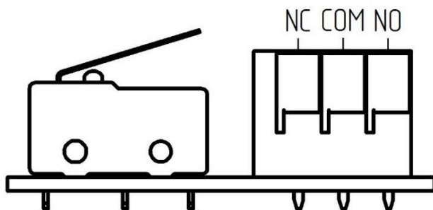
Рисунок 8.1 – Схема подключения
