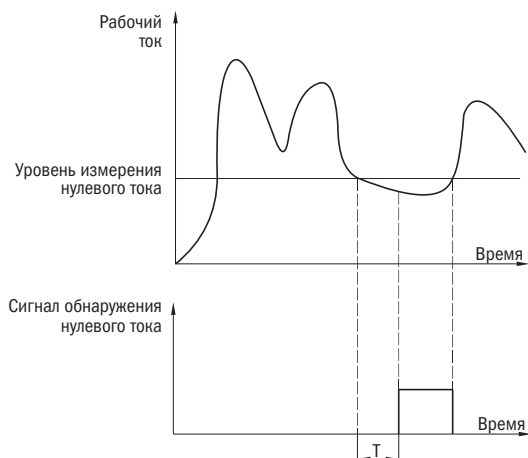
Рисунок 37 – Измерение нулевого тока
