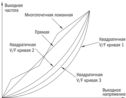
Рисунок 29 – V/F-кривые
