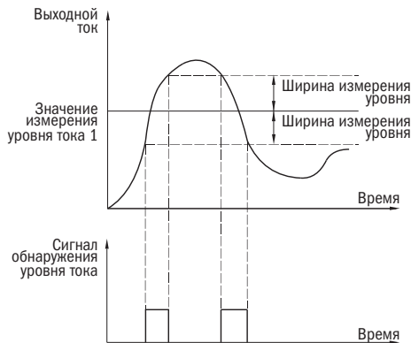
Рисунок 39 – Измерение уровня тока
