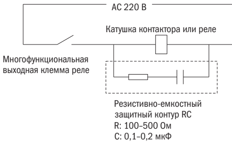
Рисунок 16 – Подключение выходного реле на переменный ток
