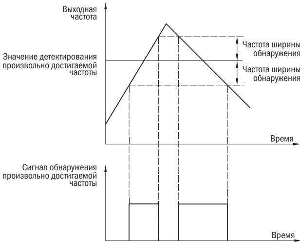
Рисунок 36 – Произвольно достигаемая частота
