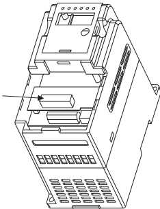
Рисунок В.8 – Место подключения платы расширения
