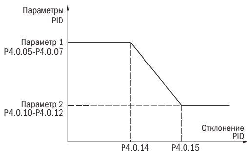
Рисунок 40 – Переключение ПИД
