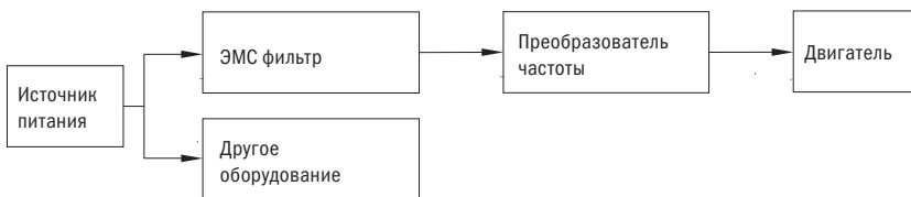
Рисунок 11 – Подключение фильтра со стороны входа
