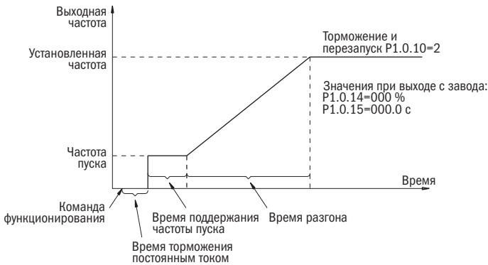
Рисунок 54 – Пуск с торможением постоянным током
