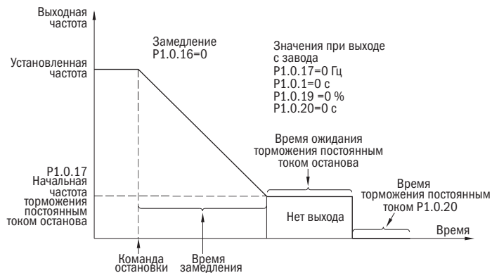
Рисунок 55 - Остановка замедлением
