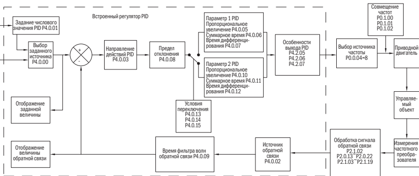
Рисунок 59 – Структура ПИД-регулятора
