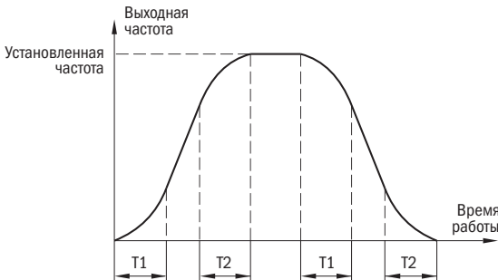
Рисунок 27 – Соотношение S-кривых
