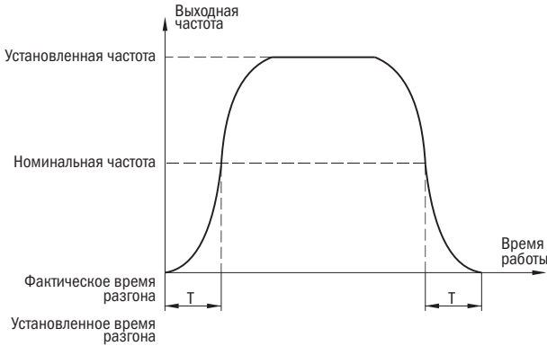
Рисунок 26 – S-кривая ускорения и замедления
