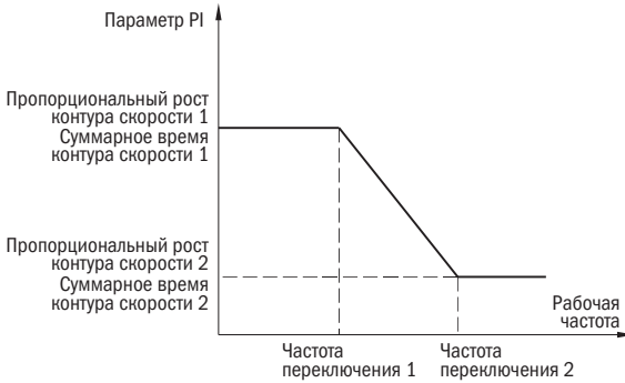
Рисунок 30 – Частоты переключения
