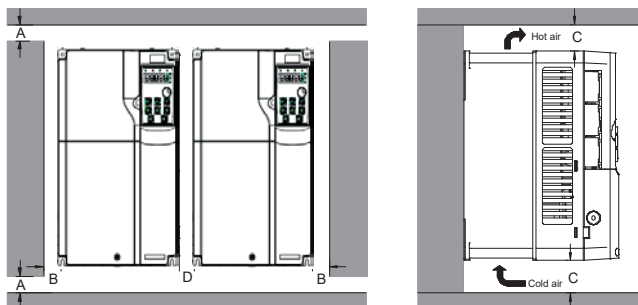
Рис. 4-4 Параллельная установка
