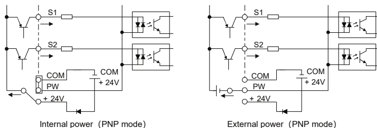
Рис. 4–32 PNP режим
