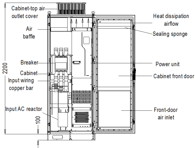
Рис. 4-7 Схема монтажа ПЧ в шкаф с прямым выпуском
