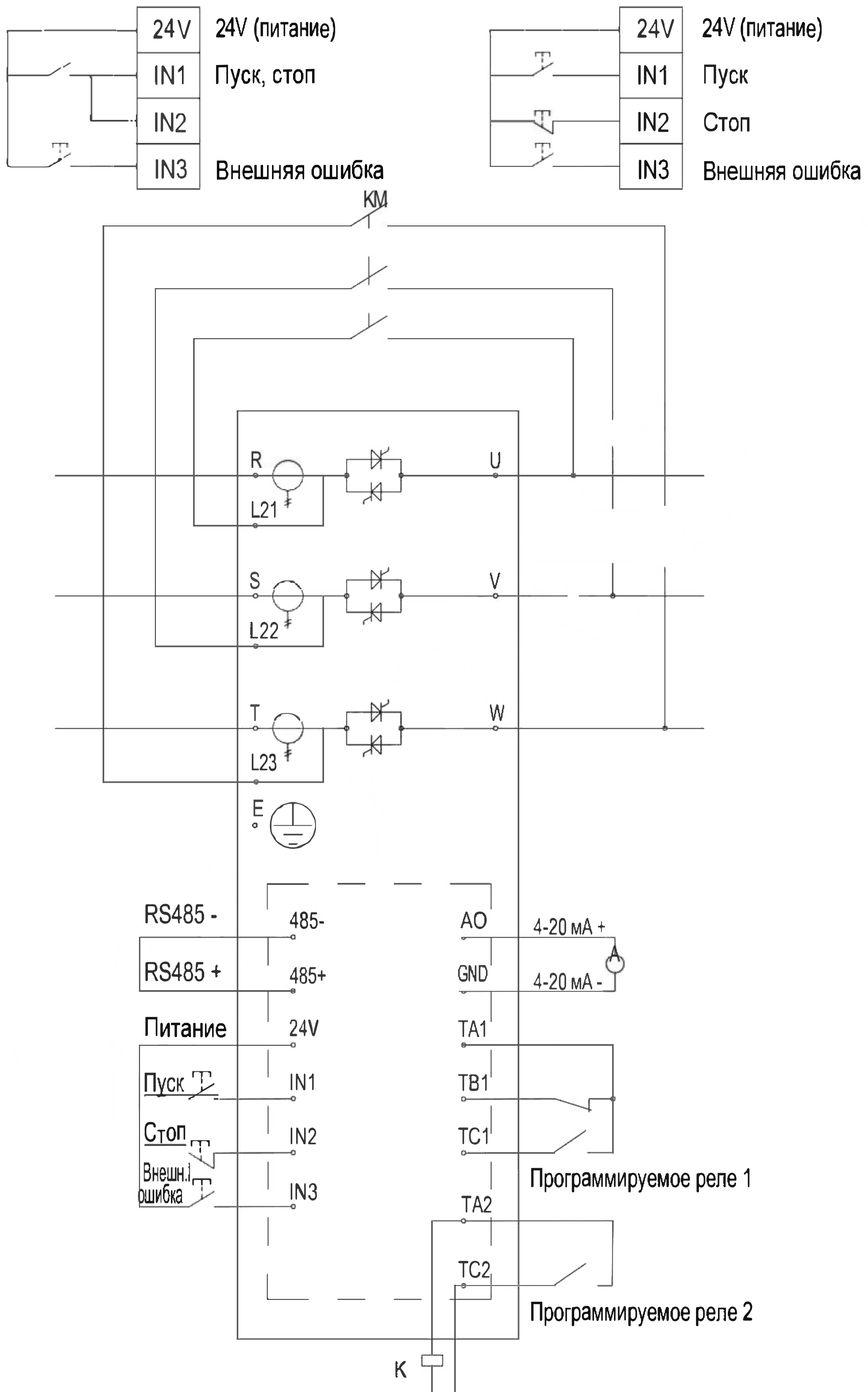
Двухпроводная схема
