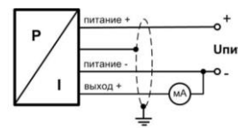
3-проводная линия (вых. сигнал - ток)
