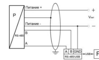
4-х проводная линия (интерфейс RS-485)
