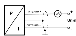
2-проводная линия (вых. сигнал - ток)
