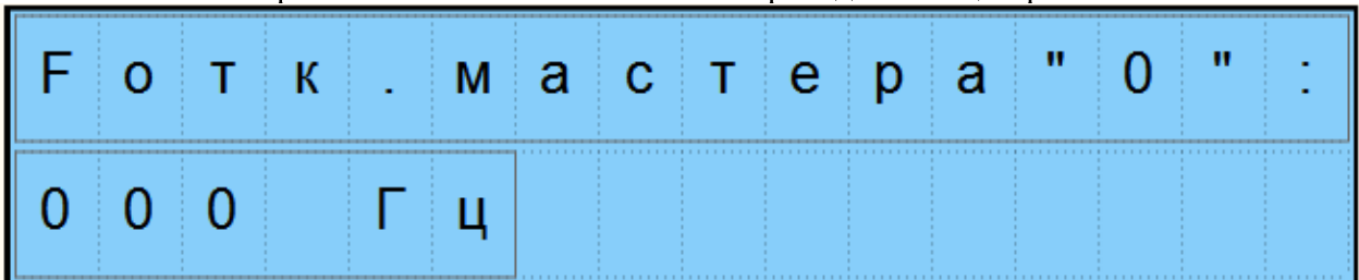
Экран частоты основного насоса перехода в спящий режим
