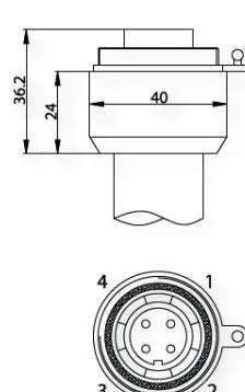
Разъем Bussaneer, 4-конт. / IP 68
