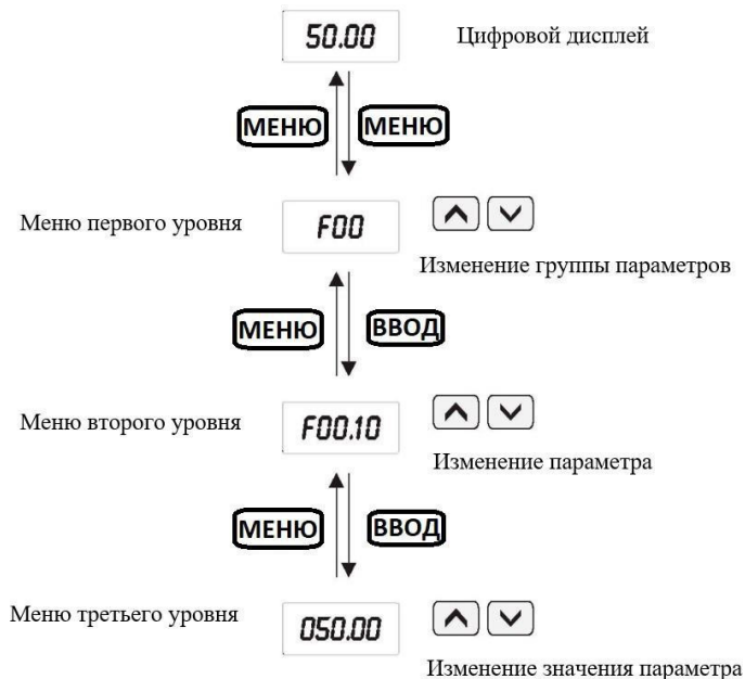
Рисунок 6.1 – Схема настройки параметров меню
