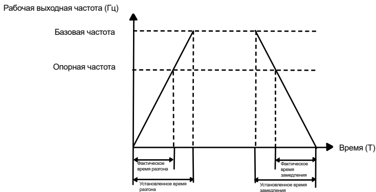
Рисунок 6.2 – Время разгона/замедления
