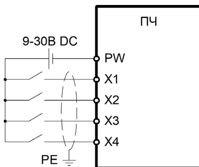
Рисунок 3.18 – Схема подключения, при которой используется внешний источник питания, цифровые входы в режиме PNP
