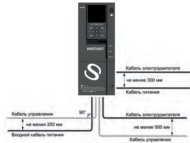
Рис. 3.6 Графическое представление расстояний между кабелями
