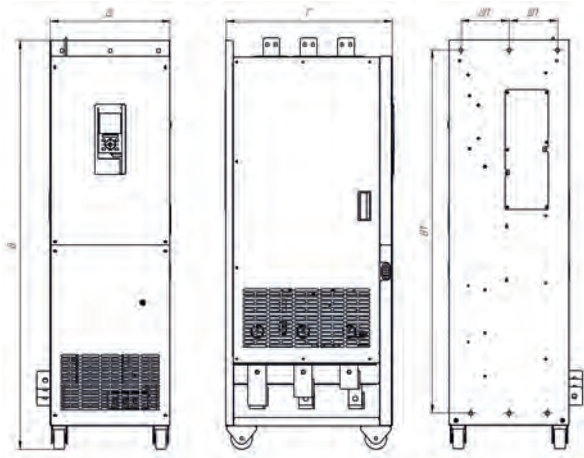
Рис 2.5. Габаритные и установочные размеры ПЧ серии INPRIME типоразмеров 9-10
