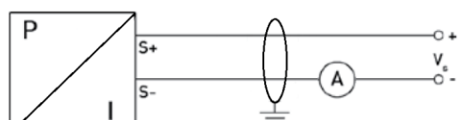
2-х проводная линия (выходной сигнал - ток)
