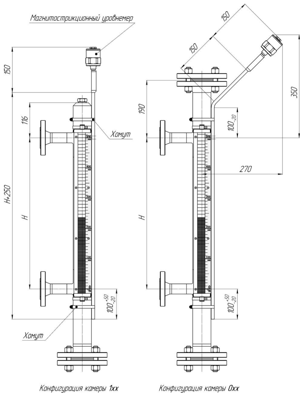
Рисунок 7.4 – Общий вид указателя уровня модельных групп ILL-BM-B16 / -B40 с магнитоэлектрическим уровнем
