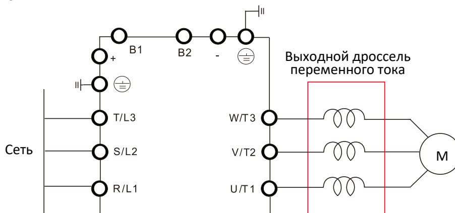
Подключение выходного дросселя
