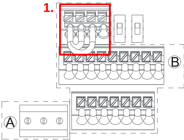
Расположение клемм управления
