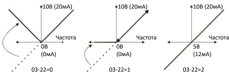
Выходной аналоговый сигнал в зависимости от направления вращения
