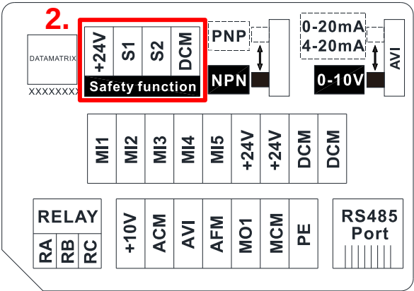
Назначение клемм управления
