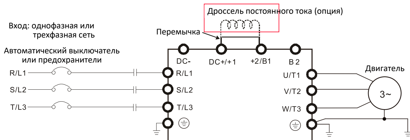
Подключение дросселя постоянного тока
