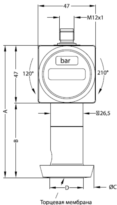
Торцевая мембрана
