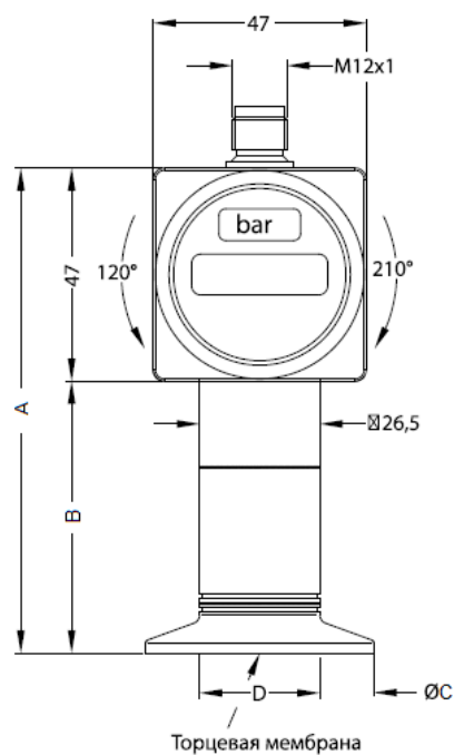
Торцевая мембрана
