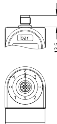
Код N00 или N10 (Разъем M12x1, 5-конт. / IP 67 или разъем M12x1 металлический, 5-конт. / IP 67)
