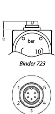
Код 200 (Разъем Binder 723, 5-конт. / IP 67)
