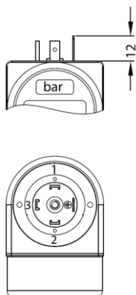
Код 100 (Разъем DIN 43650 (ISO 4400) / IP 65)
