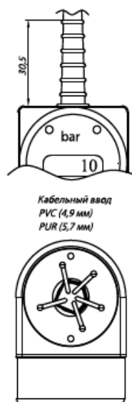
Код TR0 (Герметичный каб. ввод для погружного исполнения с кабелем PVC 4 м / IP 68)
