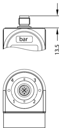
Код M00 или M10 (Разъем M12x1, 4-конт. / IP 67 или разъем M12x1 металлический, 4-конт. / IP 67)
