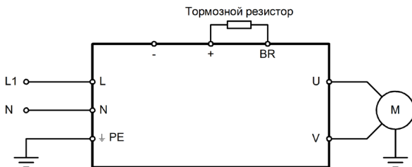
Рисунок 3.2 – Схема силовых подключений для моделей NCI-GY/PY-1B
