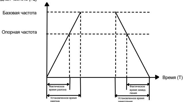
Рисунок 6.3 – Время разгона/замедления
