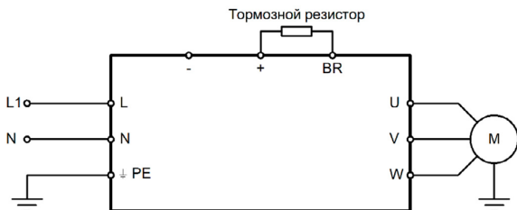
Рисунок 3.3 – Схема силовых подключений для моделей NCI-GY/PY-2B
