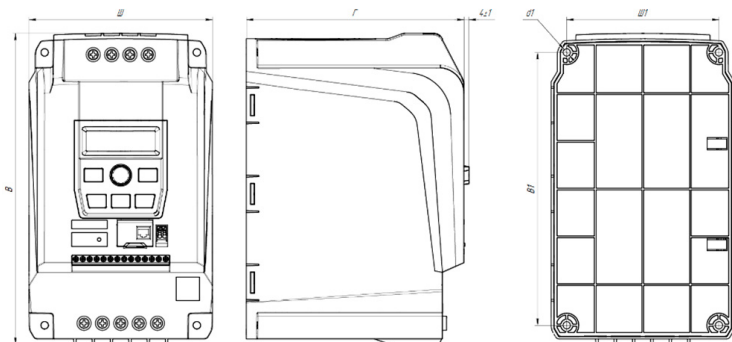
Рисунок 2.6 – Габаритные и установочные размеры устройств серии NCI
