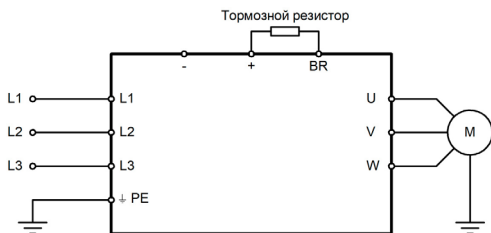
Рисунок 3.4 – Схема силовых подключений для моделей NCI-GY/PY-4B
