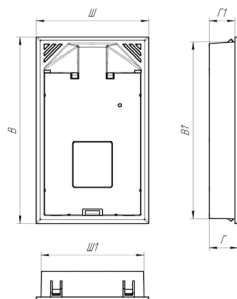
Рисунок 5.3 – Монтажный комплект NCI-MK и монтажная рамка NCI-MF
