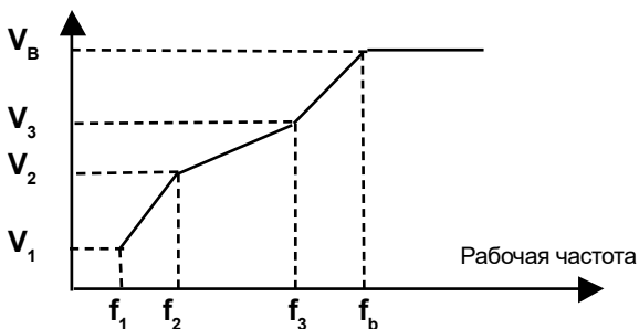
Рисунок 6.7 – Ломаная характеристика V/f
