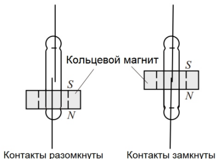
Схема срабатывания геркона
