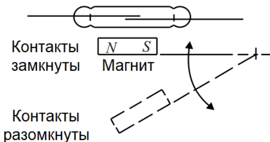
Схема срабатывания геркона
