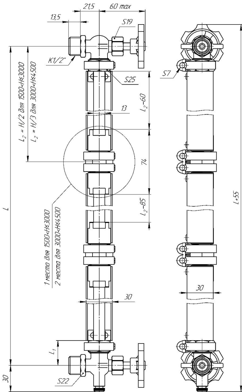
Рисунок 7.1.2 – Общий вид указателя с присоединительной длиной H > 1500 мм и наружным резьбовым присоединением K1/2"
