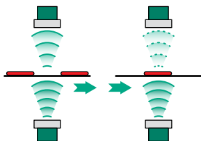
Рисунок 2 – Прохождение ультразвуковой волны через материал
