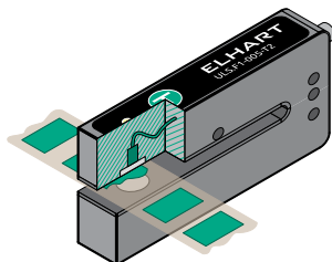
Рисунок 1 – Устройство датчика
