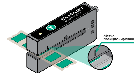
Рисунок 5 – Позиционирование
