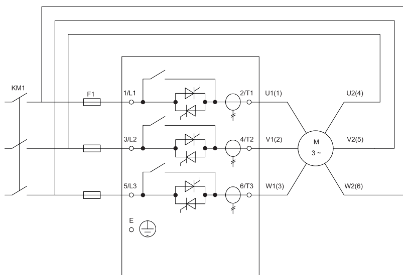
Рисунок 3.7 – Схема подключения двигателя «звезда»
