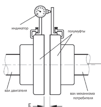
Рисунок 5 – Схема измерения аксиальной несоосности
