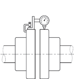
Рисунок 6 – Схема измерения радиальной несоосности (смещения осей)
