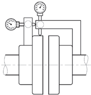
Рисунок 7 – Схема комбинированного измерения аксиальной и радиальной несоосности
