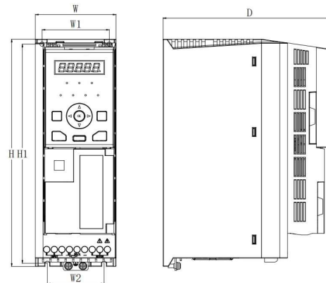
Рис. 1. IMD_E 0,75 – 5,5 кВт
