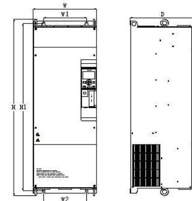
Рис. 4. IMD_E 37 – 200 кВт
