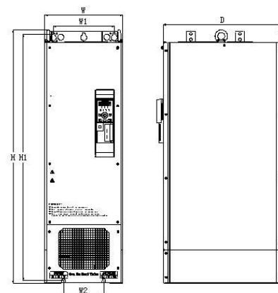
Рис. 5. IMD_E 220 – 450 кВт
