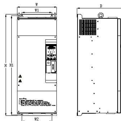
Рис. 3. IMD_E 18,5 – 30 кВт
