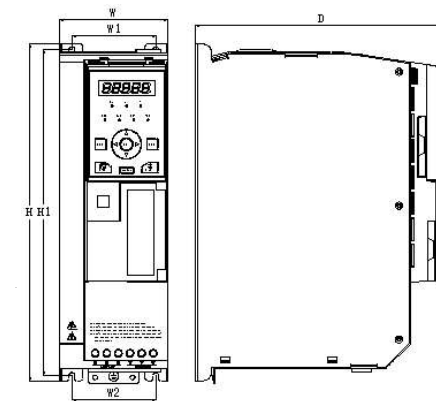
Рис. 2. IMD_E 7,5 – 15 кВт
