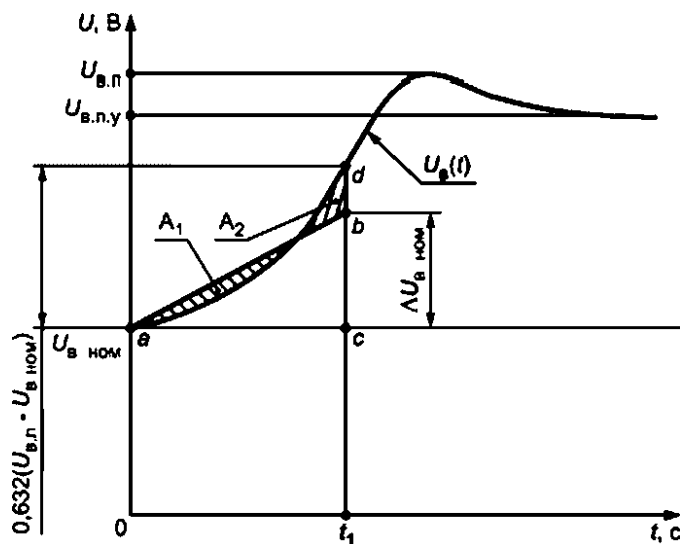
Рисунок А.1 — Определение номинальной скорости нарастания напряжения возбуждения
