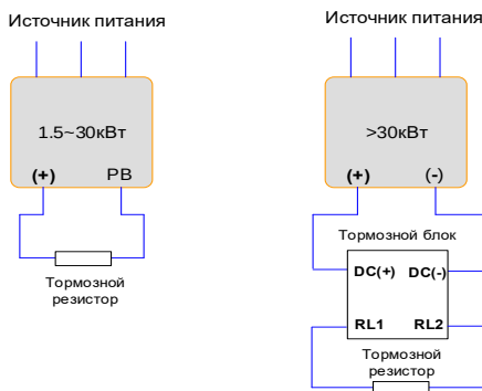
Рисунок 2-4. Схема подключения тормозной системы к преобразователю частоты до 30кВт со встроенным тормозным блоком(левая) и более 30кВт с внешним тормозным блоком(правая).
