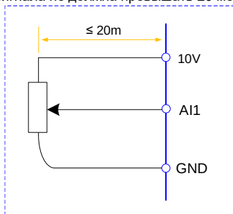
Рисунок 3-6. Схема подключения к аналоговому входу ПЧ
