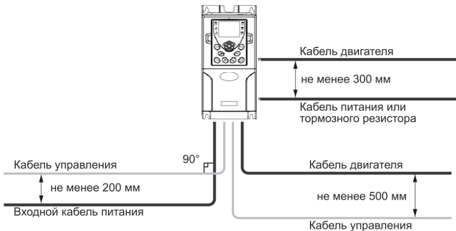
Рисунок 3-5. Схема расположения кабелей преобразователя частоты
