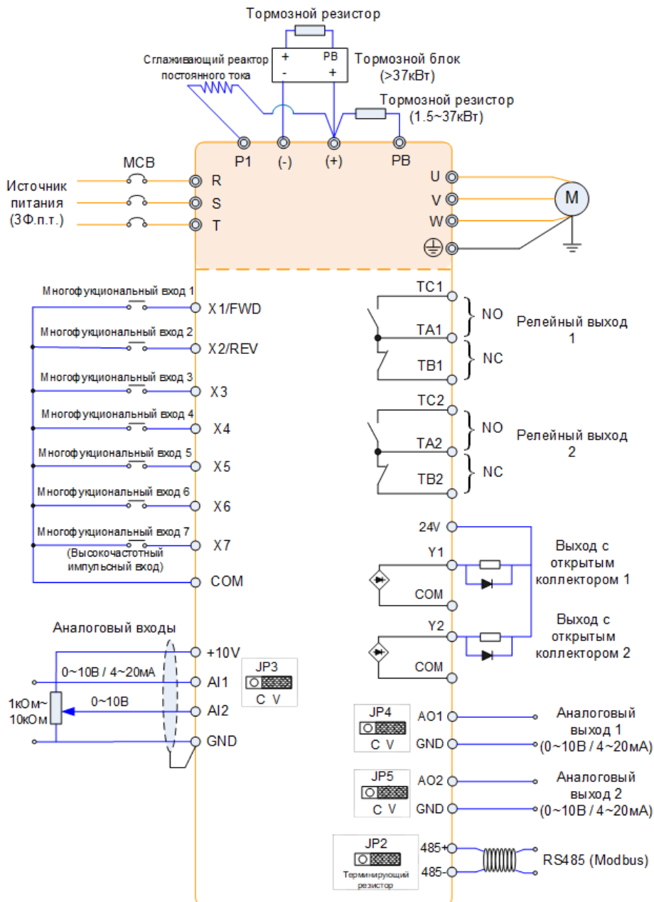
Рисунок 3-3. Принципиальная электрическая схема подключения
