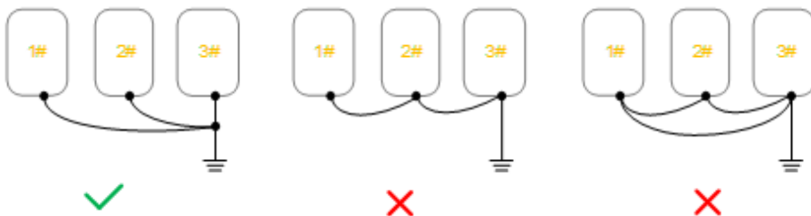
Рисунок 3-7. Схема заземления ПЧ.
