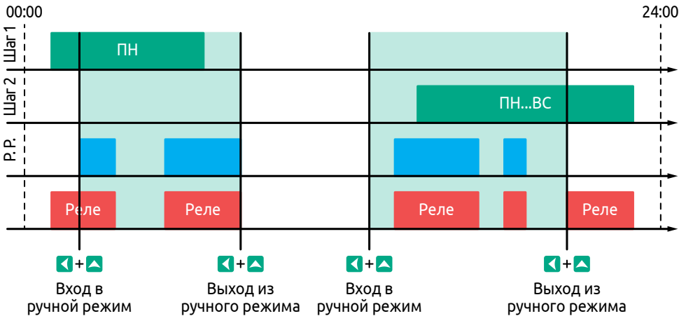
Рисунок 15 - Ручной режим
