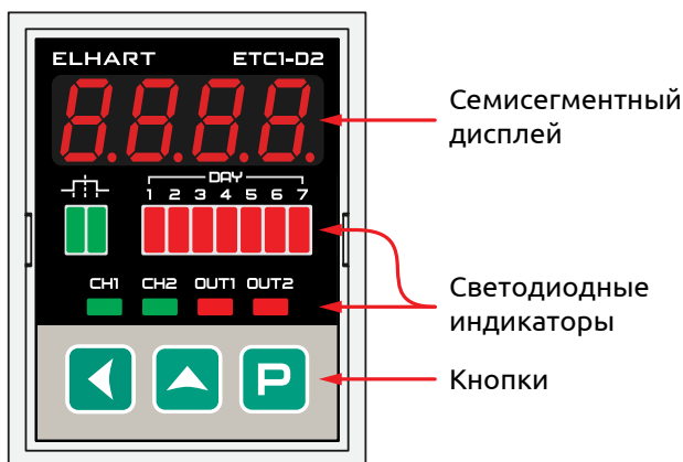
Рисунок 10 - Лицевая панель
