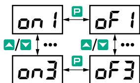
Рисунок 13 – Навигация в меню прибора
