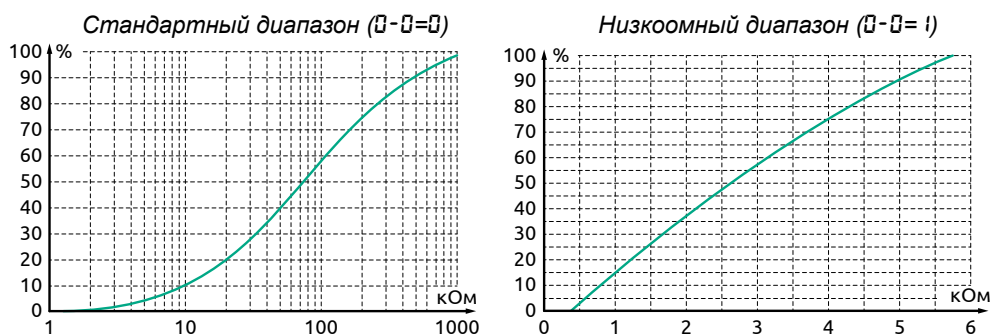
Рисунок 15 – График настройки чувствительности входов
