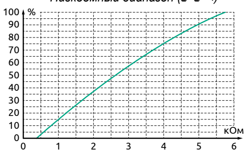
Рисунок 14 – График настройки чувствительности входов
