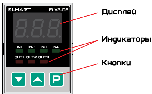
Рисунок 12 – Лицевая панель
