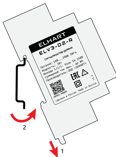
Рисунок 16 – Демонтаж прибора
