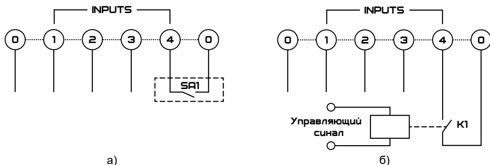
а) подключение через выключатель, б) подключение через реле
