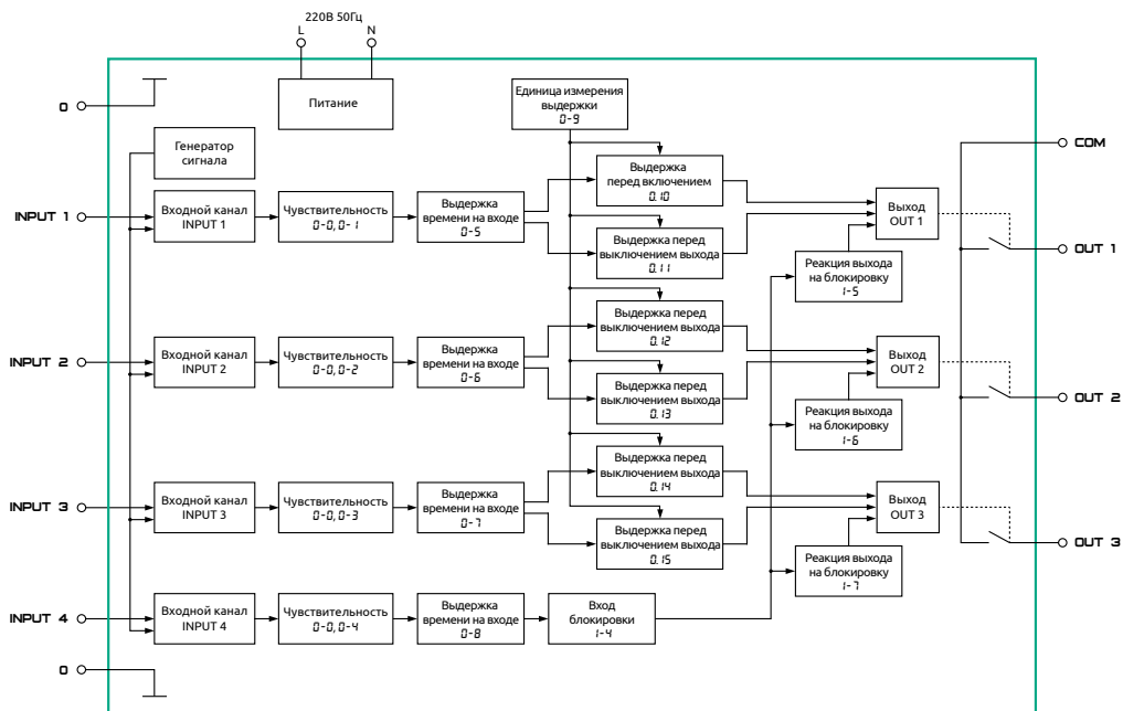
Рисунок 11 – Функциональная схема прибора
