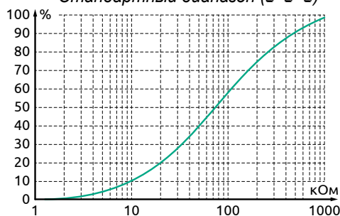
Рисунок 14 – График настройки чувствительности входов
