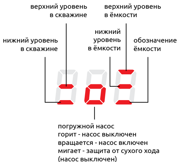
Рисунок 26 – Индикация алгоритма 1
