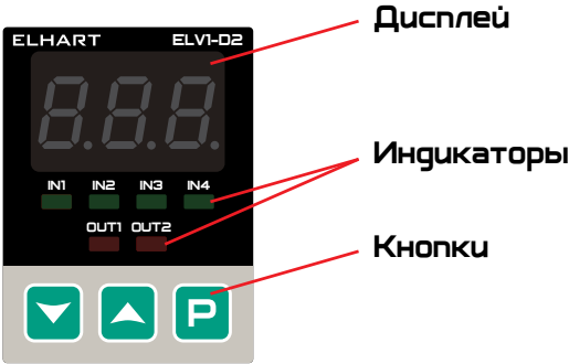
Рисунок 21 — Лицевая панель
