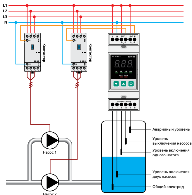
Рисунок 67 – Наполнение емкости с чередованием насосов
