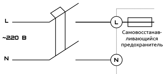
Рисунок 13 – Схема подключения напряжения питания
