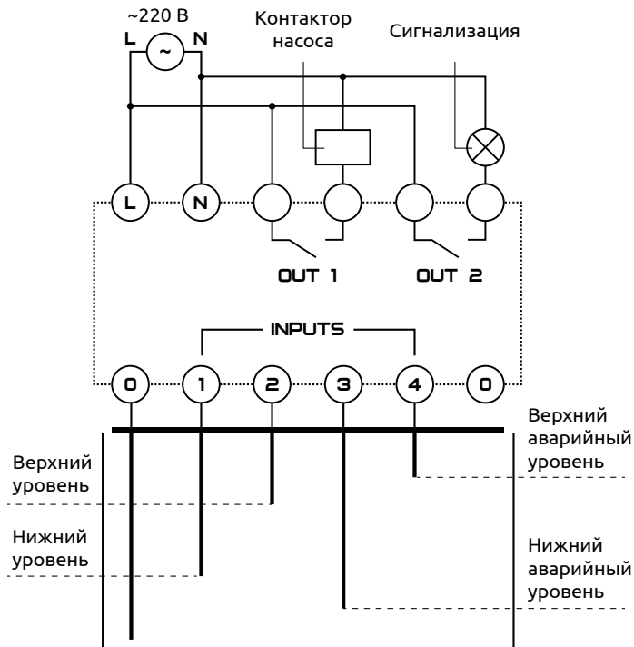
Рисунок 27 – Схема подключения для алгоритма 2
