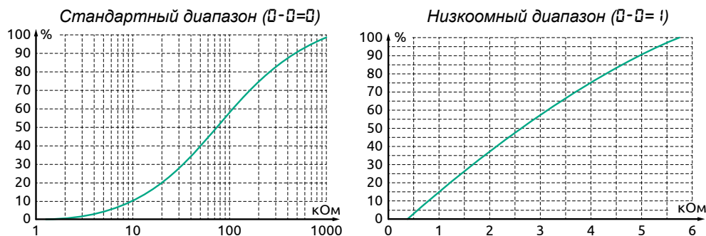
Рисунок 23 – График настройки чувствительности входов
