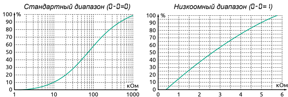
Рисунок 36 – График настройки чувствительности входов
