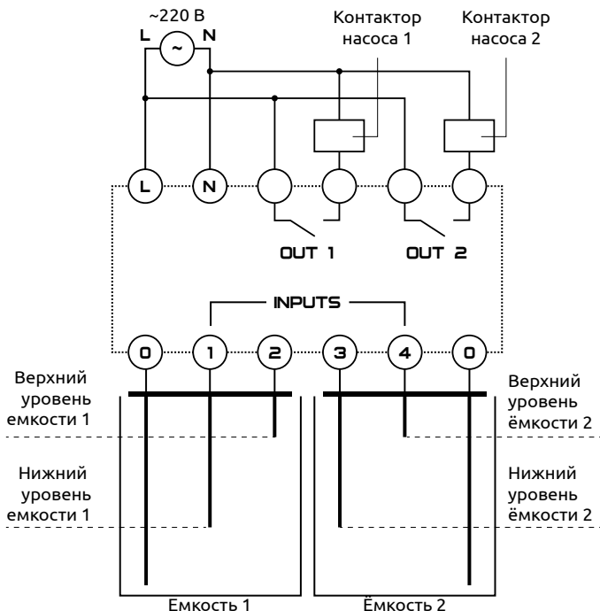
Рисунок 9 – Схема подключения для алгоритма 3
