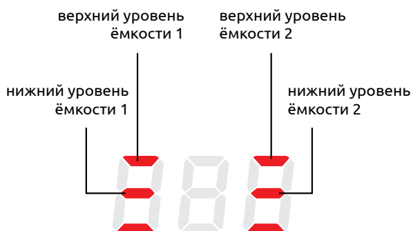
Рисунок 32 – Индикация алгоритма 3
