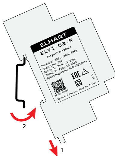
Рисунок 41 – Демонтаж прибора
