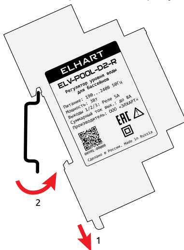
Рисунок 15 – Демонтаж прибора
