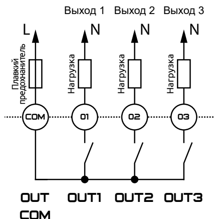
Рисунок 9 — Схема подключения выходов
