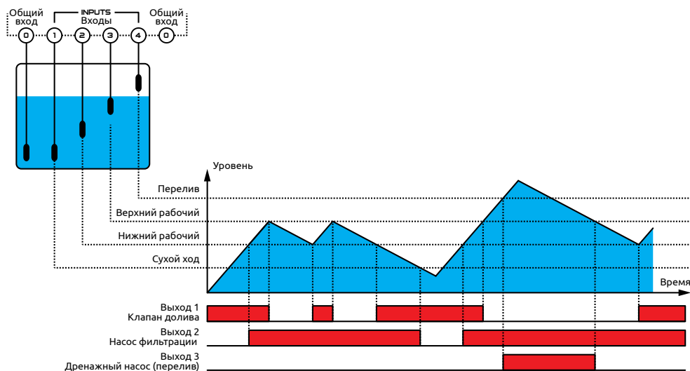
Рисунок 11 – Диаграмма работы выходов
