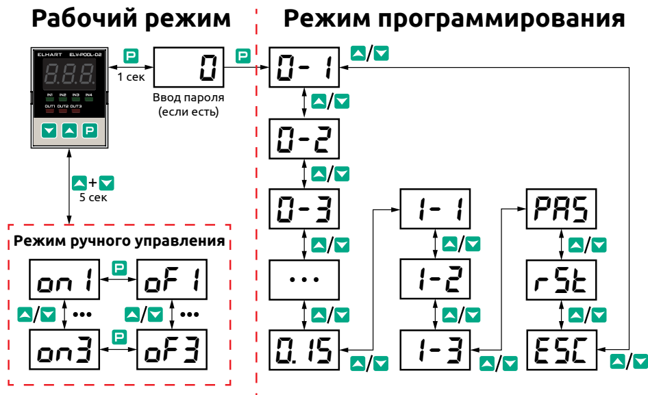
Рисунок 13 – Навигация в меню прибора
