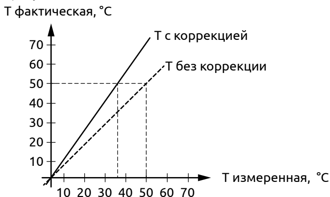
Рисунок 26 - Наклон характеристики измерительного входа
