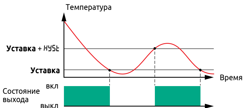
Рисунок 17 - Работа двухпозиционного регулятора в режиме «Холодильник»
