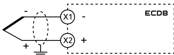
Рисунок 6 - Схема подключения термопар
