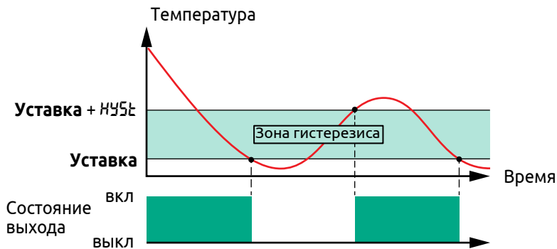
Рисунок 23 - Работа двухпозиционного регулятора в режиме «Холодильник»
