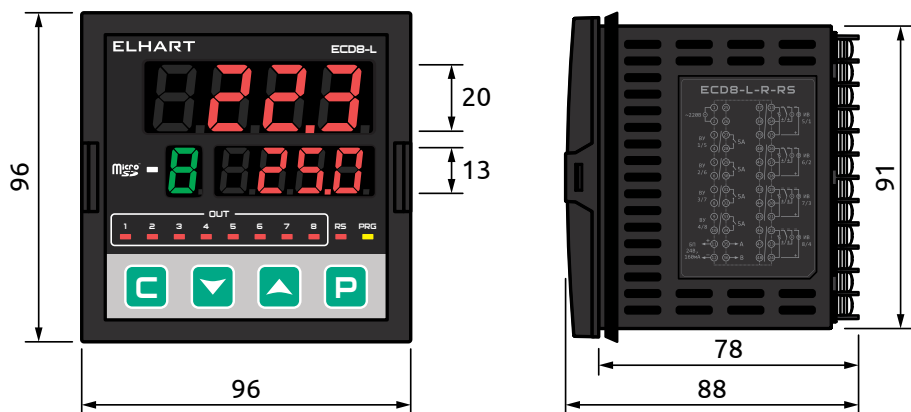
Рисунок 1 - Внешний вид и основные размеры прибора
