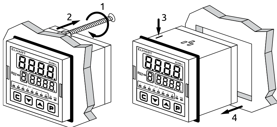
Рисунок 31 - Демонтаж прибора
