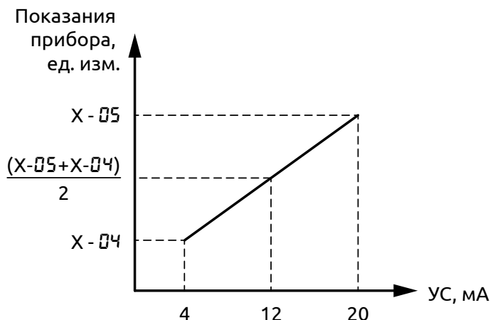
Рисунок 25 - Масштабирование диапазона датчиков с унифицированным сигналом 4 \dots 20 мА
