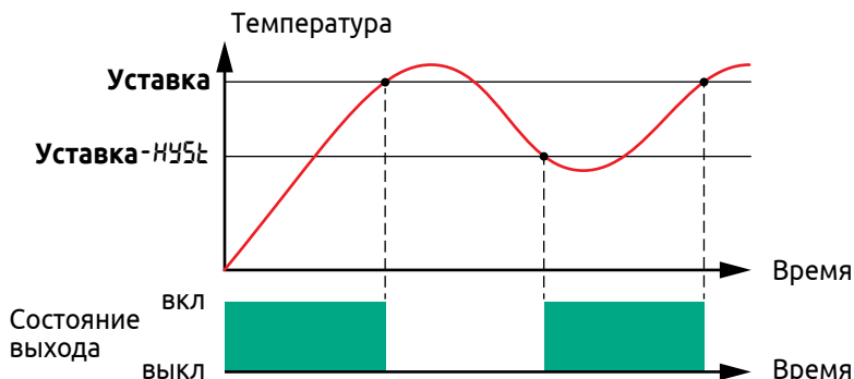
Рисунок 16 - Работа двухпозиционного регулятора в режиме «Нагреватель»
