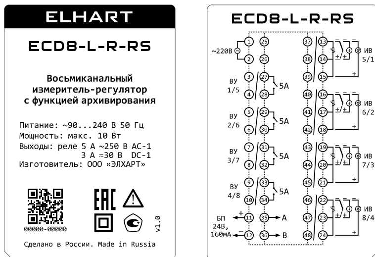
Рисунок 32 - Маркировка прибора
