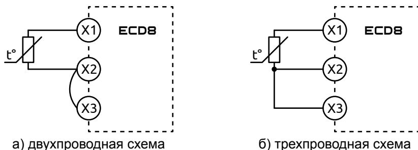
Рисунок 7 - Схема подключения термосопротивления
