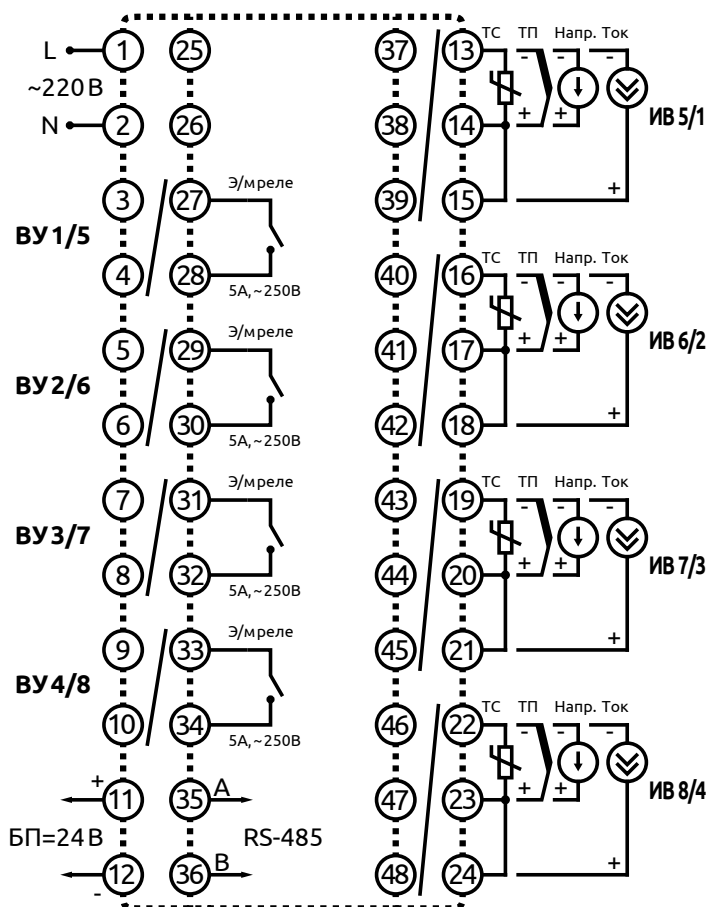
Рисунок 3 - Схема внешних соединений
