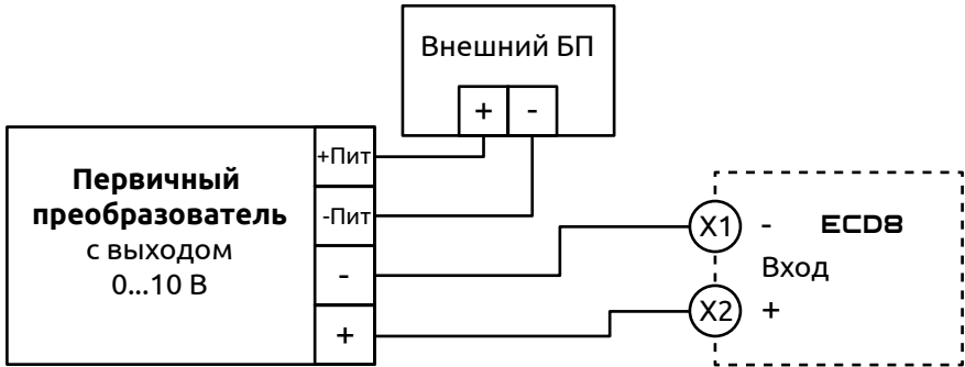
Рисунок 11 - Схема подключения первичного преобразователя с унифицированным сигналом напряжения и с использованием внешнего блока питания
