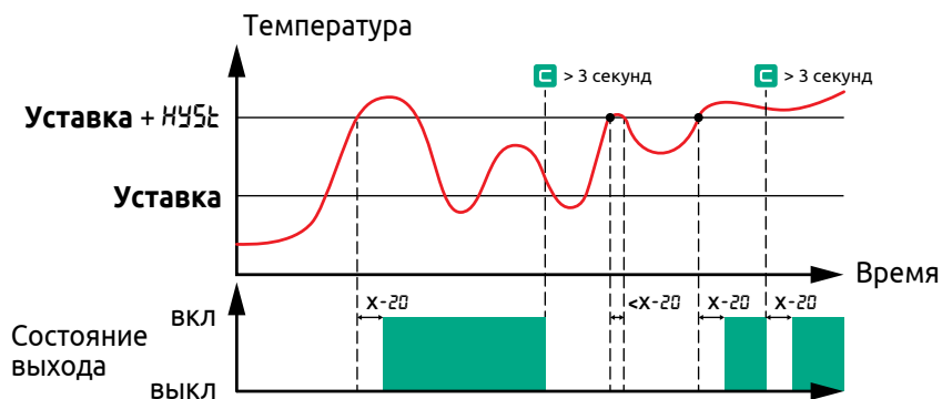
Рисунок 21 - Работа выхода при включенной фиксации
