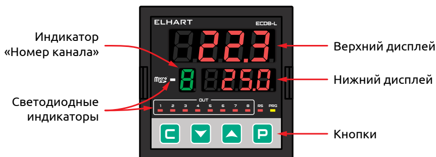
Рисунок 14 - Лицевая панель
