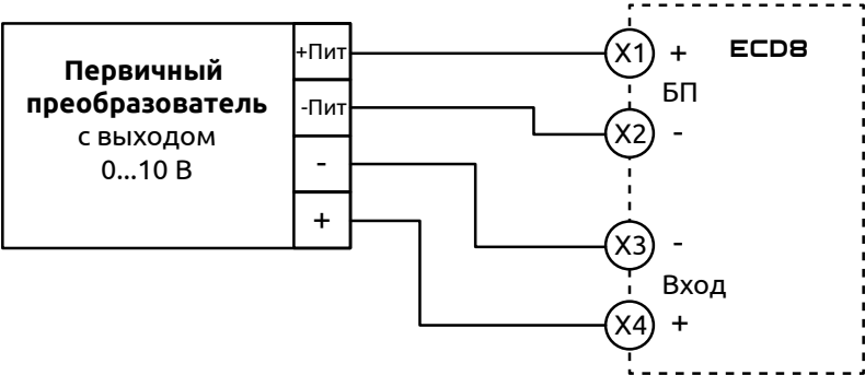
Рисунок 10 - Схема подключения первичного преобразователя с унифицированным сигналом напряжения с использованием встроенного блока питания
