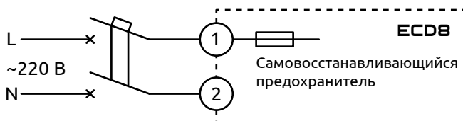
Рисунок 4 - Схема подключения напряжения питания
