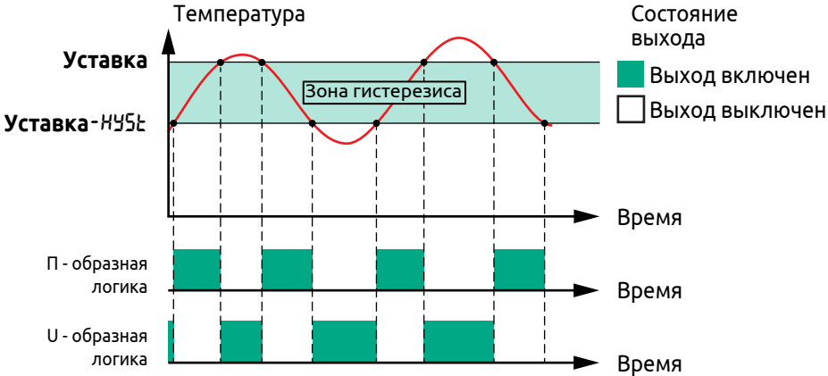
Рисунок 24 - Работа сигнализатора
