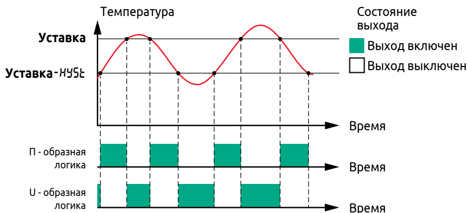
Рисунок 19 - Работа сигнализатора
