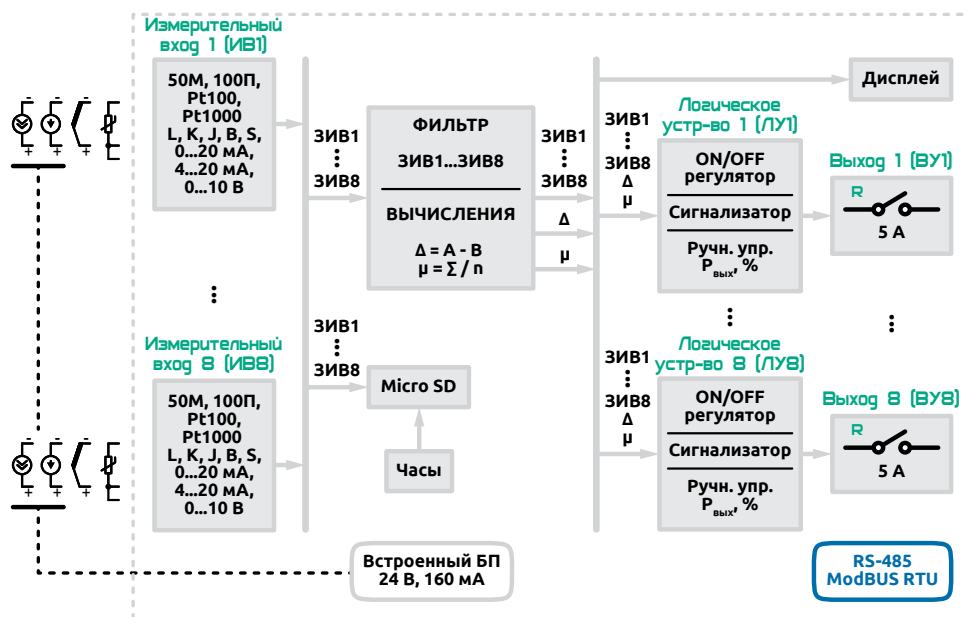
Рисунок 13 - Функциональная схема прибора
