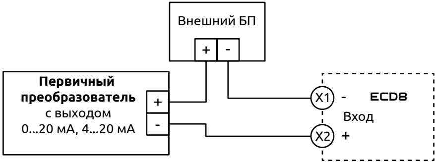
Рисунок 9 - Схема подключения первичного преобразователя с унифицированным сигналом тока с использованием внешнего блока питания
