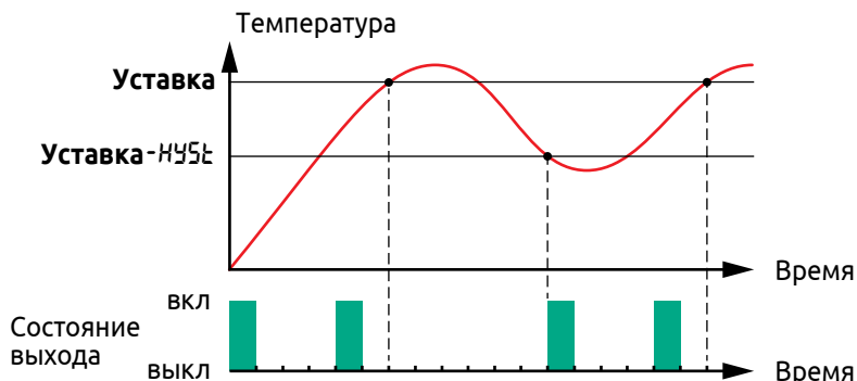
Рисунок 29 - Ограничение выходного сигнала двухпозиционного регулятора в режиме «нагреватель»
