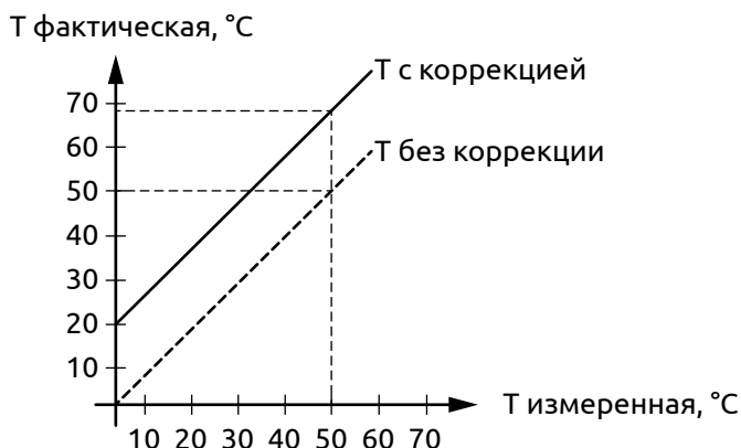
Рисунок 27 - Сдвиг характеристики измерительного входа
