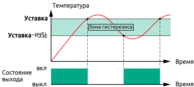
Рисунок 22 - Работа двухпозиционного регулятора в режиме «Нагреватель»
