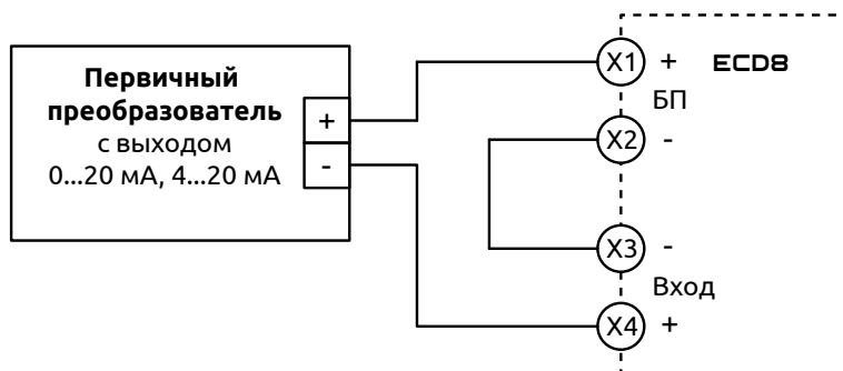
Рисунок 8 - Схема подключения первичного преобразователя с унифицированным сигналом тока с использованием встроенного блока питания
