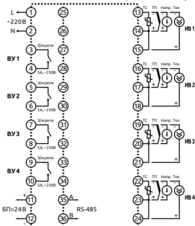
Рисунок 3 - Схема внешних соединений ECD4-L-R
