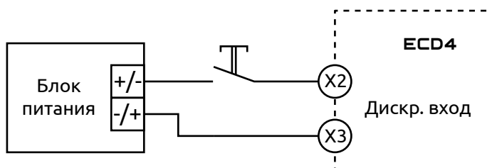
Рисунок 14 - Схема подключения кнопки «сухой контакт» с использованием блока питания к дискретным входам прибора
