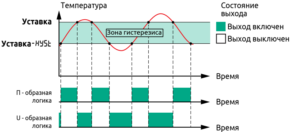
Рисунок 29 - Работа сигнализатора
