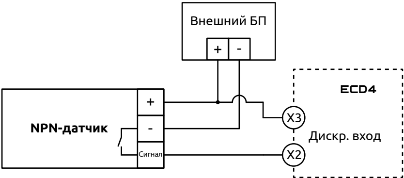
Рисунок 16 - Схема подключения NPN-датчиков к дискретным входам прибора
