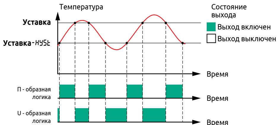
Рисунок 24 - Работа сигнализатора
