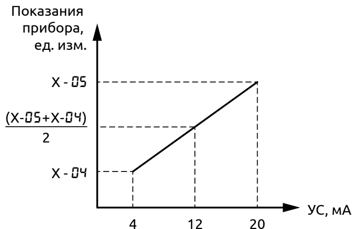
Рисунок 30 - Масштабирование диапазона датчиков с унифицированным сигналом 4...20 мА
