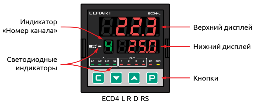
Рисунок 19 - Лицевая панель
