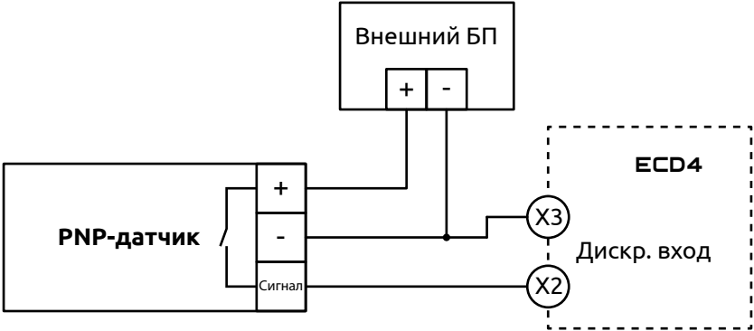
Рисунок 15 - Схема подключения PNP-датчиков к дискретным входам прибора
