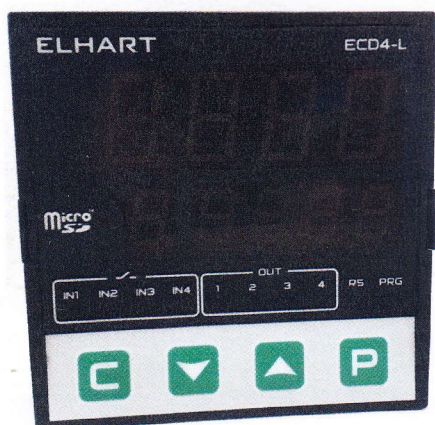
Рисунок 3 - Общий вид ECD4-L
