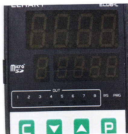
Рисунок 4 - Общий вид ECD8-L
