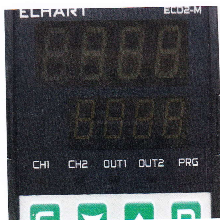
Рисунок 7 - Общий вид ECD2-M
