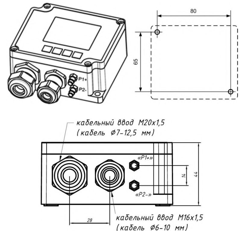
Рисунок А.1 – Вид корпуса изделия и разметка отверстий для крепления
