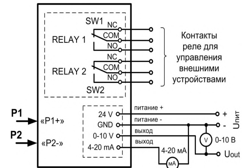
Рисунок 1 – Схема подключений, где P1, P2 – входное давление измеряемой среды (вход P1+ для более высокого, а P2– для более низкого)
