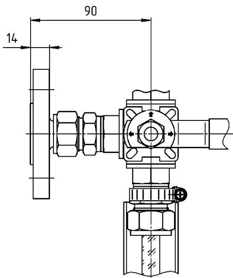
Рисунок 7.1.3 – Общий вид указателя с присоединительным фланцем Ду15 (остальное – см. рисунки 7.1.1 – 7.1.2)
