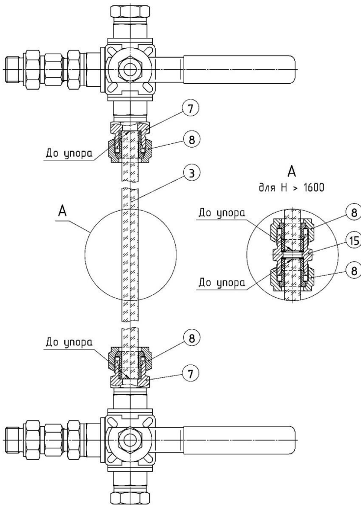
Рисунок 8.2.1 – Схема сборки смотровой трубки с фитингами
